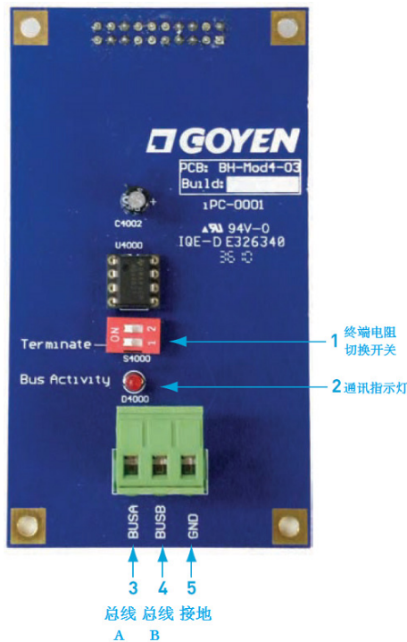
RS485 MODBUS 通讯卡
