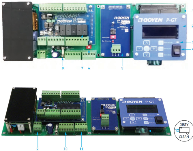
PGT-ACDC 主控制器模块
