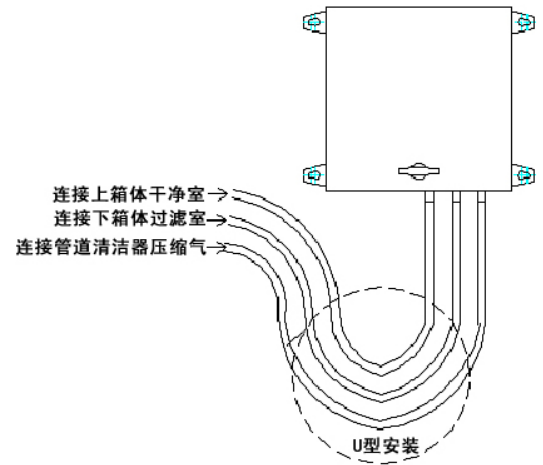
压力输送管安装图
