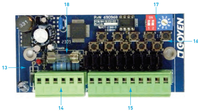
PS-C 付板控制输出模块 (24VDC 输出)
